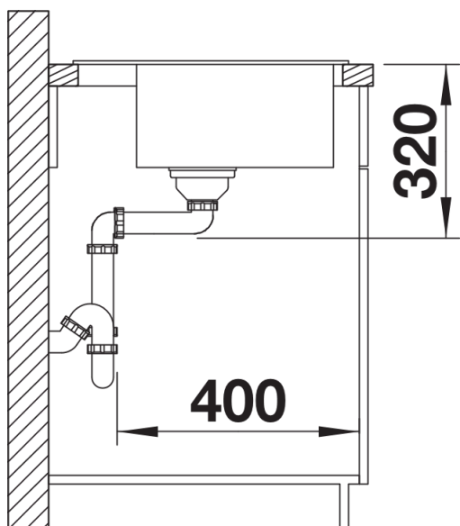
Вид сбоку
