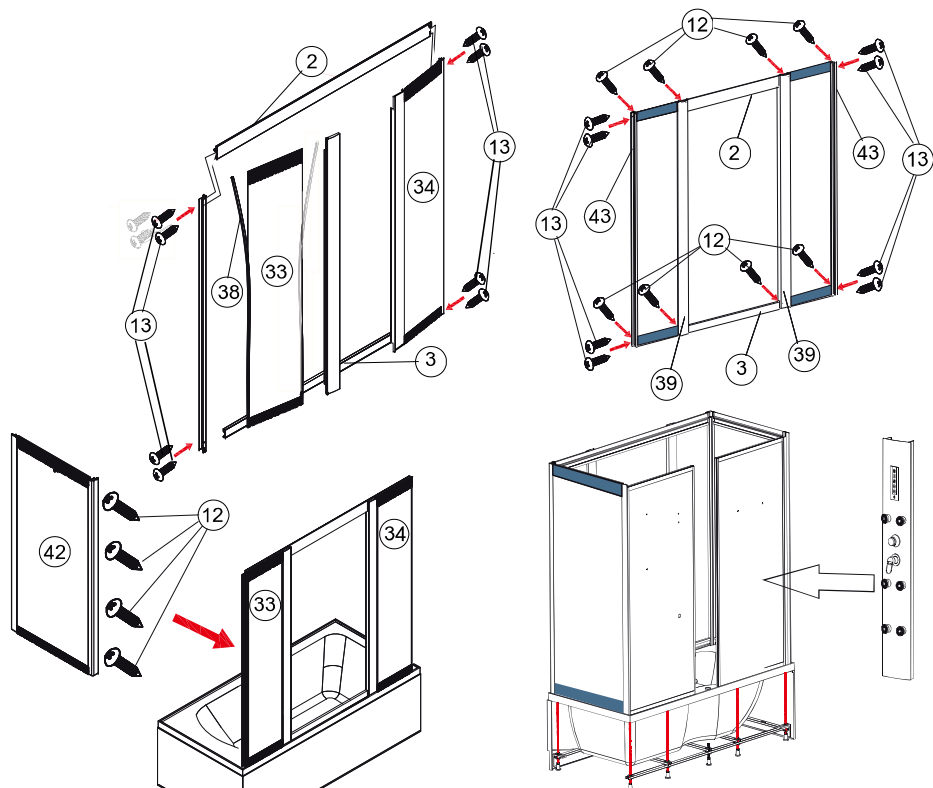
Схема установки верхней панели
