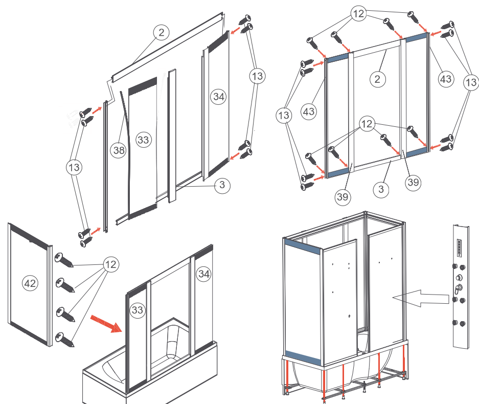
Схема установки верхней панели
