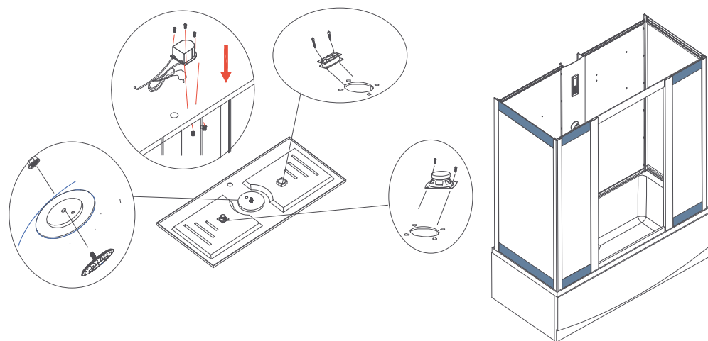
Схема установки верхней панели
