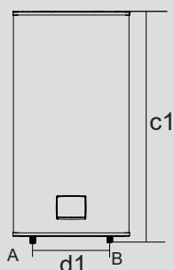
Вид спереди
