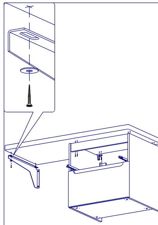
Крепление кронштейна к столешнице
