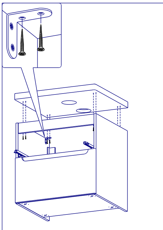
Крепление столешницы к тумбе
