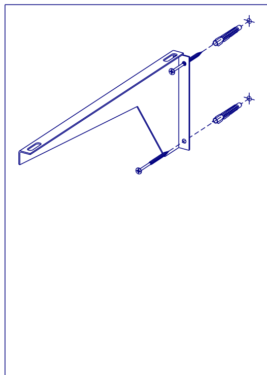
Крепление кронштейна к стене
