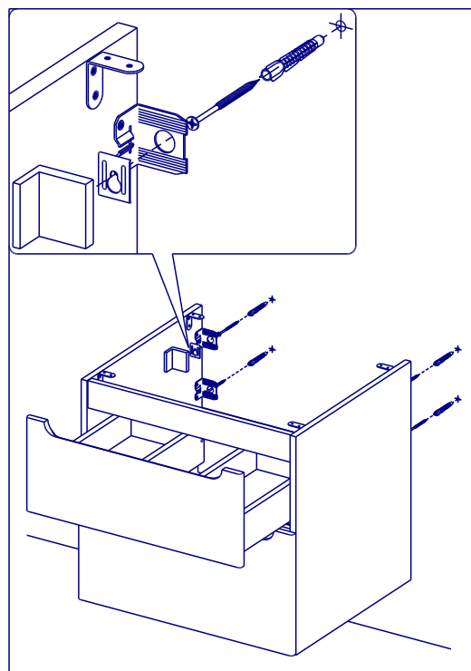
Крепление тумбы к стене
