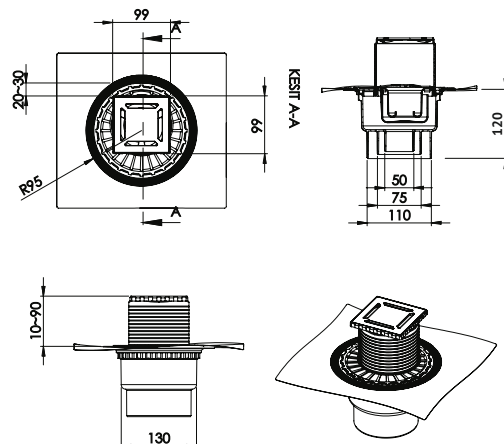
Вертикальный сифон D50/75/110 - H120 мм
