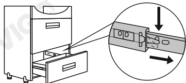
Схема зняцця шуфляды
