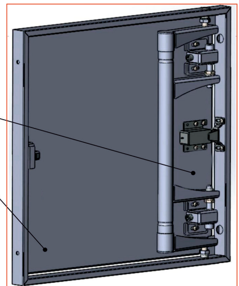
Рис. 3 Схема закрывания
