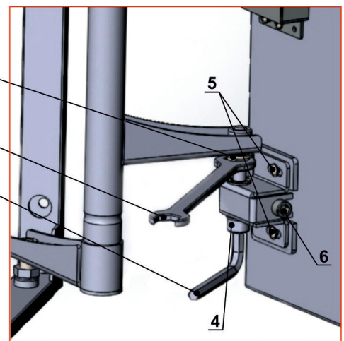
Рис. 2 Регулировка люка
