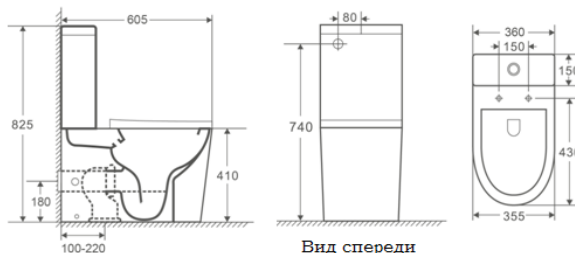
Вид спереди
