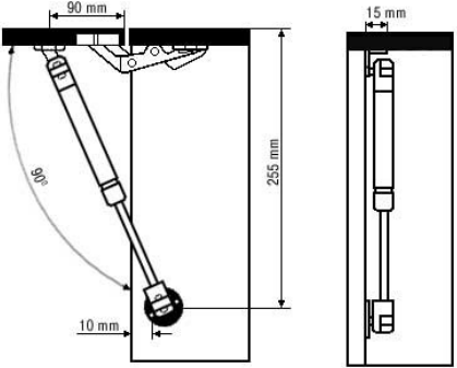
Рис.4 Установка газлифта
