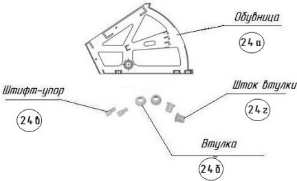
Рис.5 Комплект механизма обувницы
