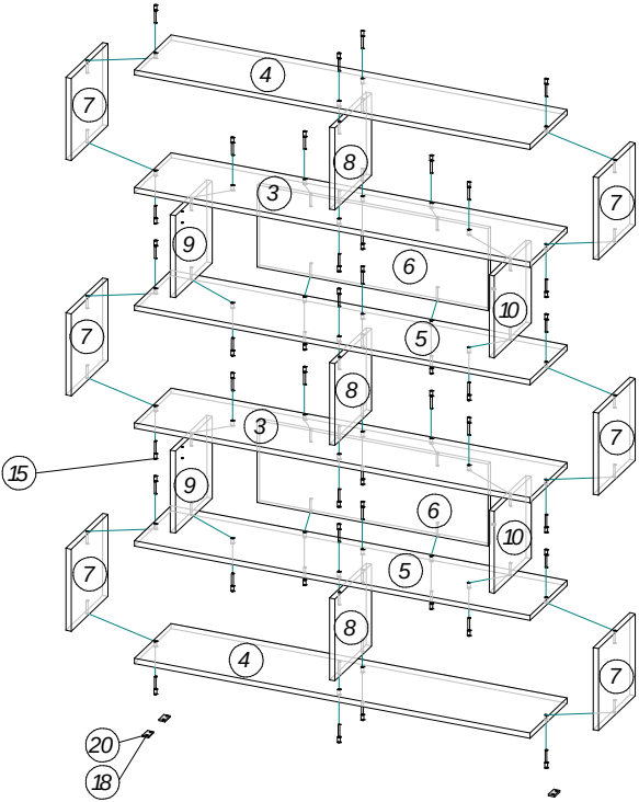
Рис.1 Сборка корпуса стеллажа
