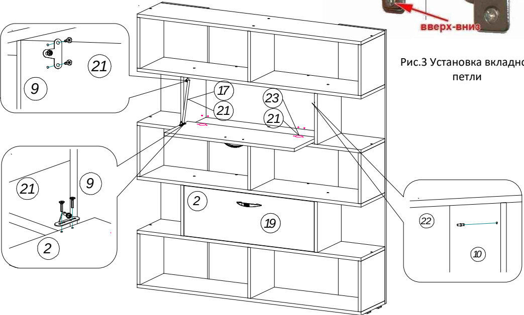
Рис.4 Установка газлифта и полкодержателя
