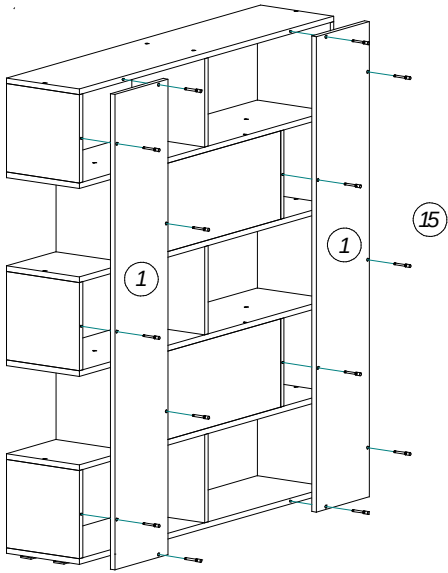
Рис.2 Установка задних стоек
