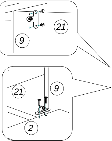
Рис.1 Сборка корпуса стеллажа
