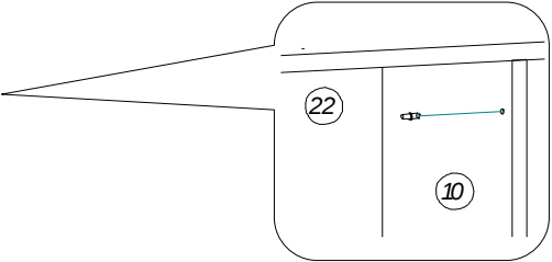
Рис.4 Установка газлифта и полкодержателя
