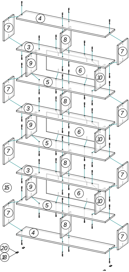
Рис.1 Сборка корпуса стеллажа
