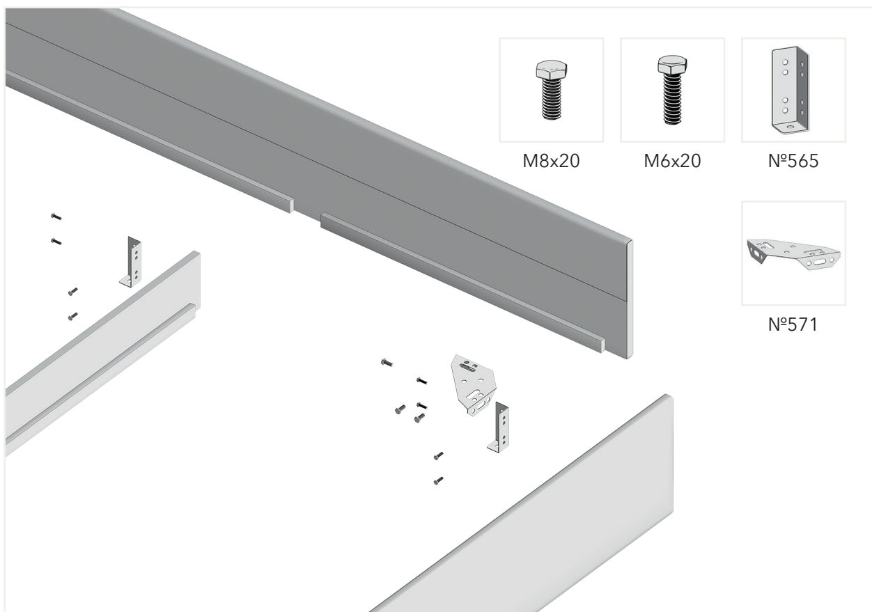
1.1.2 Соедините царги с помощью кронштейна №571 (болты M8x20) и уголка №565 (болты M6x20).
