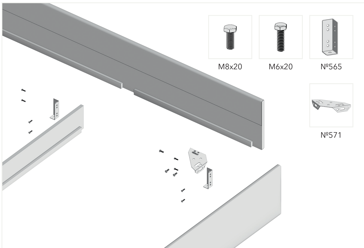
1.1.2 Соедините боковые царги и фронтальную царгу с помощью кронштейна №571 (болты M8x20, 3 шт) и уголка №565 (болты M6x20, 8 шт).
