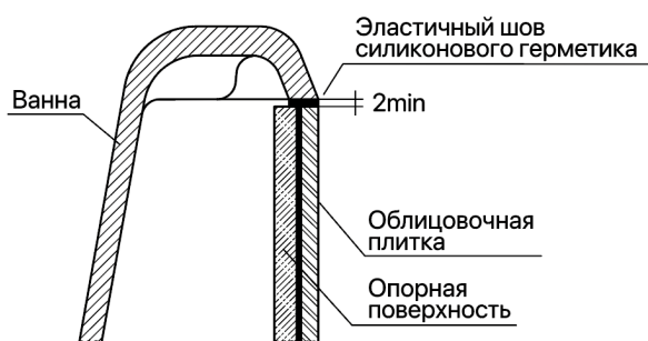
Монтаж ванны в короб, облицованный плиткой
