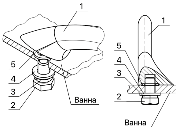
Крепление ручек
