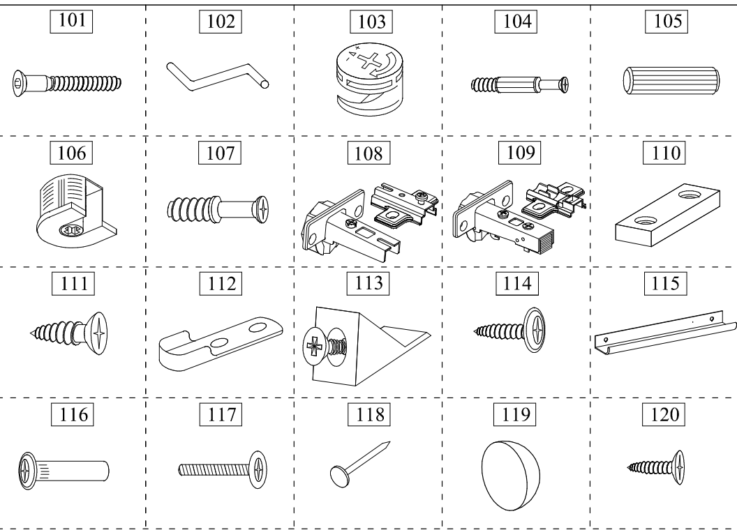
Ведомость фурнитуры
