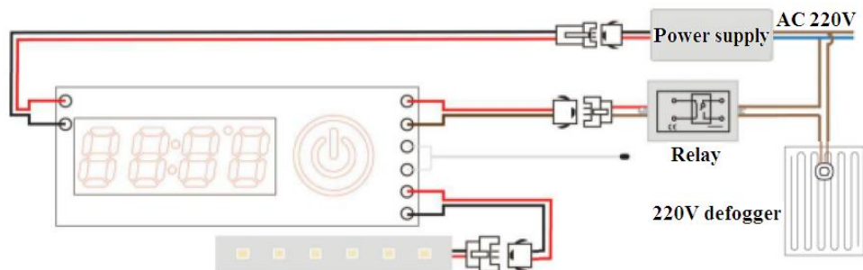
Схема подключения D12TOA-03-CTR
