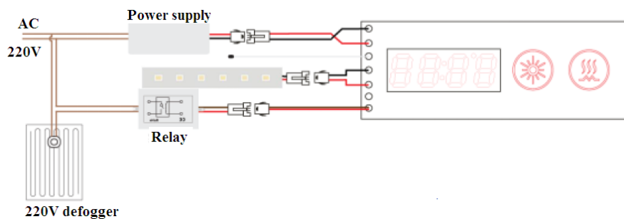
Схема подключения D12TOB-03-DCT
